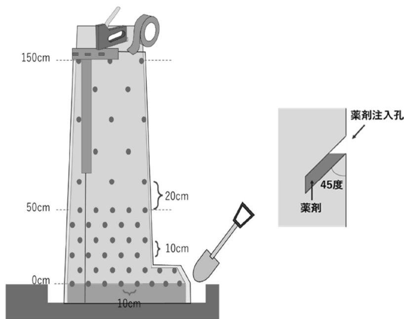
図3 立木くん蒸の模式図と薬剤注入孔の断面図
