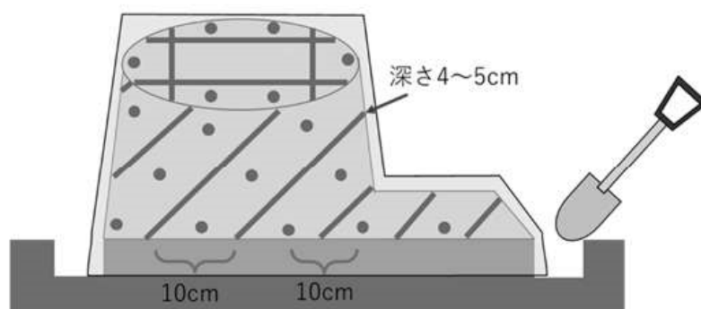
図4 伐根の処理の模式図
