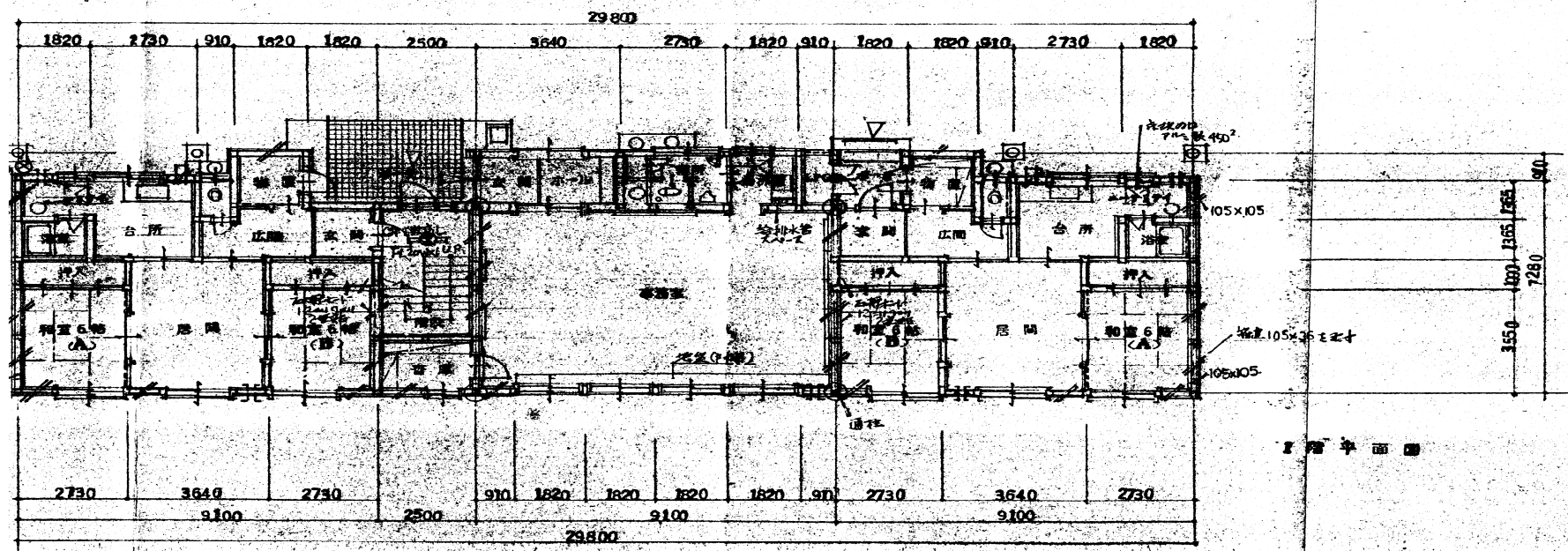
2 階 平 面 図
