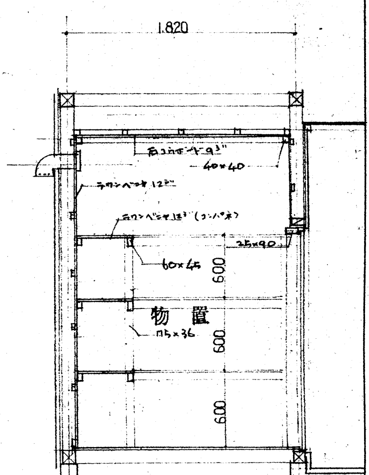
物置詳細図
