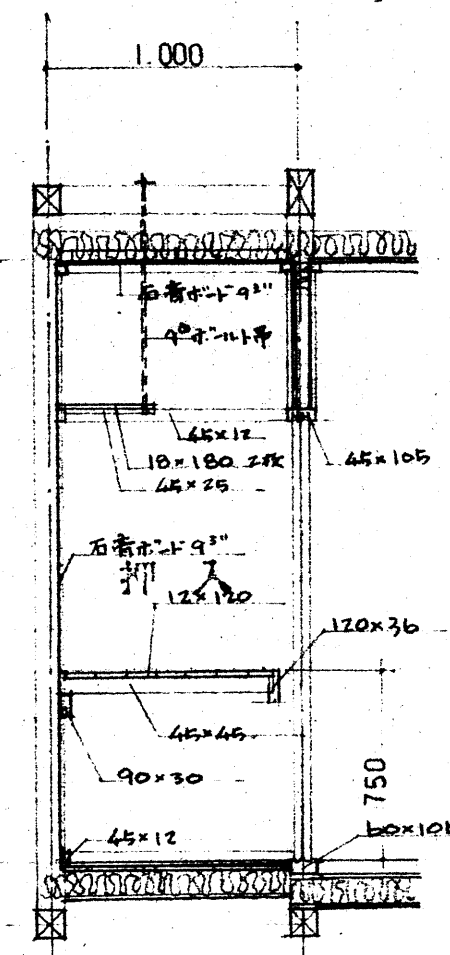
押入詳細図
