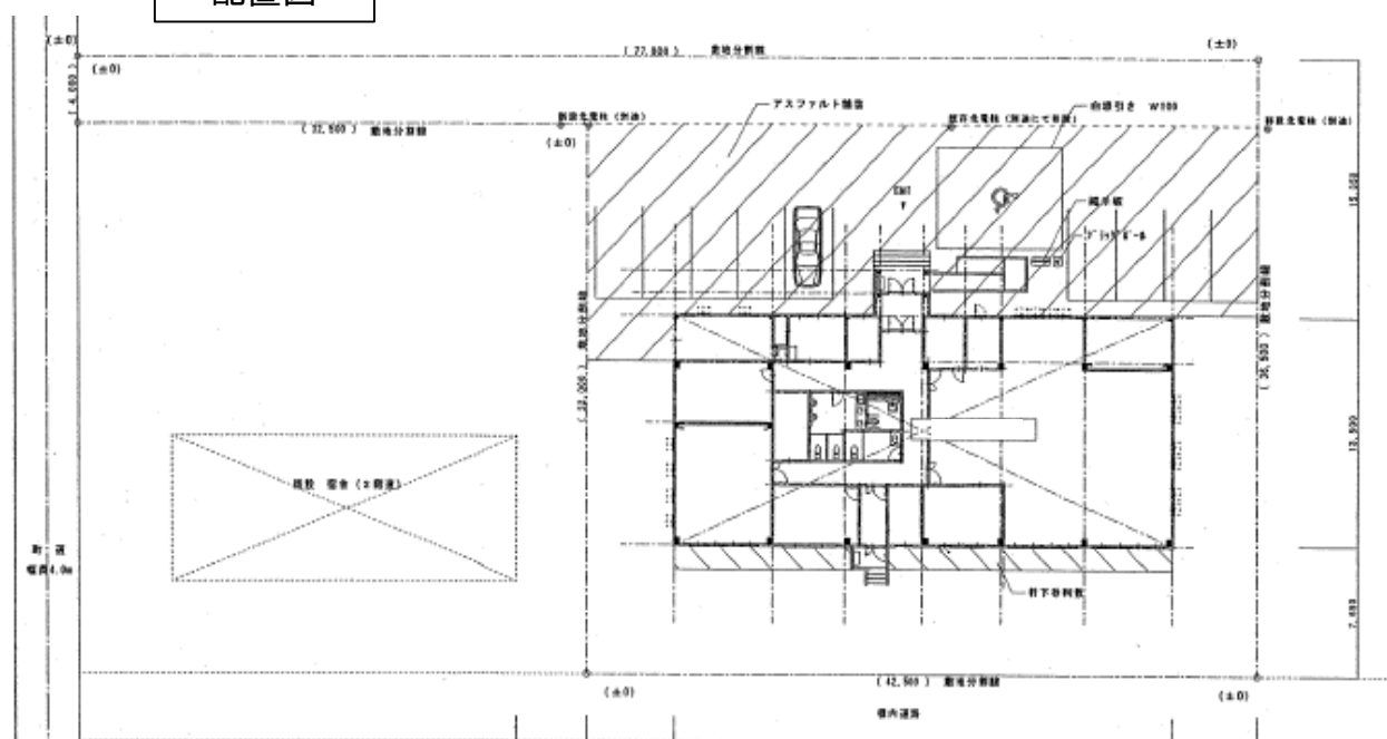
配置図
