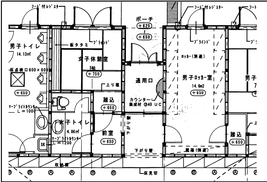
庁舎現状図面
