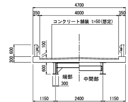
断面図 S=1:50
