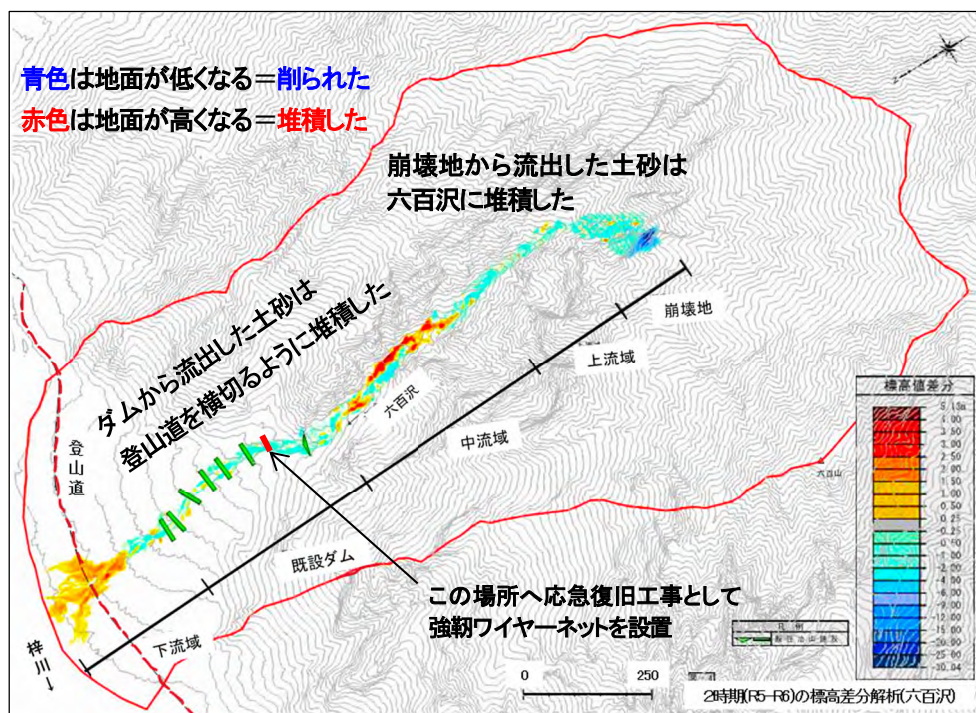
航空レーザ計測で取得したデータによる差分解析(令和6年 上高地 六百沢土石流災害箇所)
