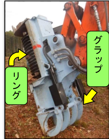
写真2：アタッチメントの写真
