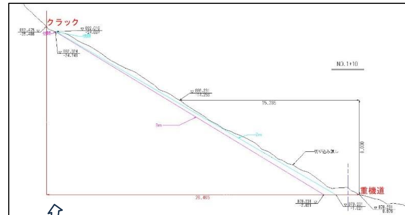
3D点群データより縦断図を作成
