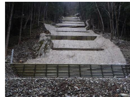
間伐材を活用した木製校倉式土留工
