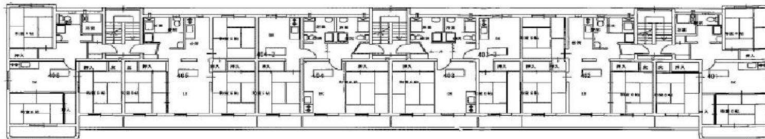
間取図（若里1号）
