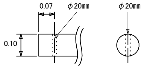
丸太詳細図
