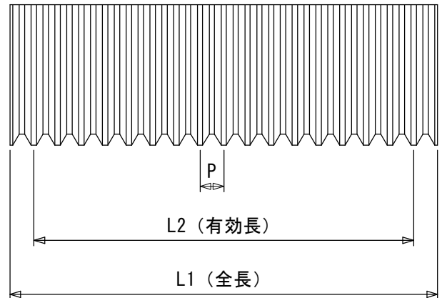
側面図
