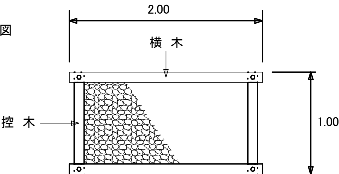
丸太詳細図
