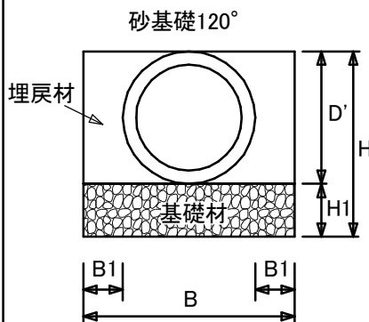
砂基礎120° 適用表及び寸法・材料表
