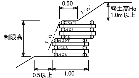
丸太詳細図
