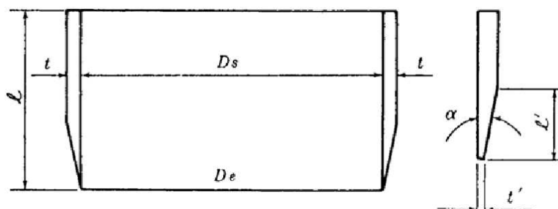
図3-1 サンプリングチューブ
