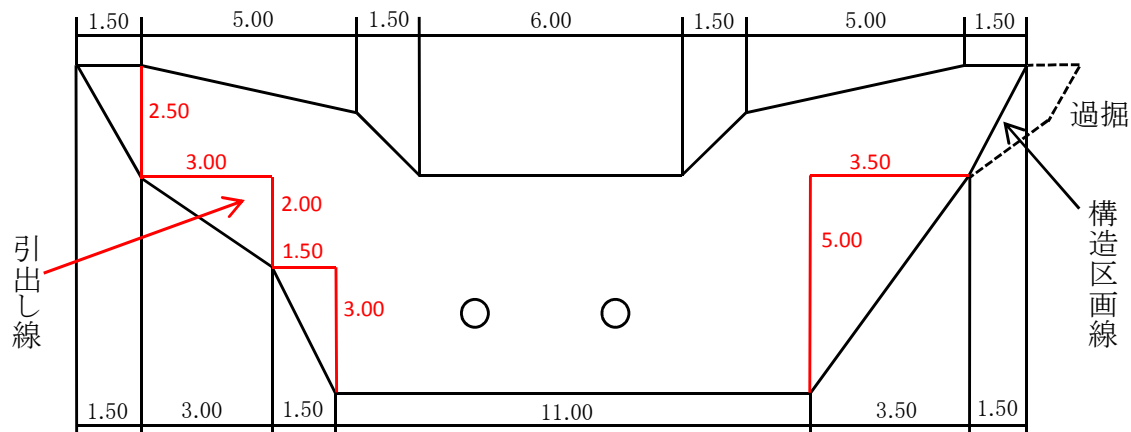
正面図
