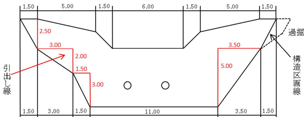
正面図
