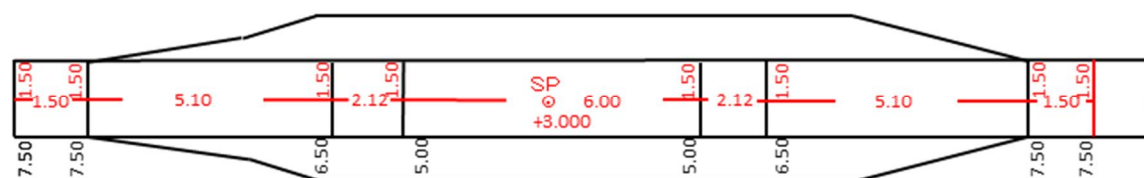
平面図
