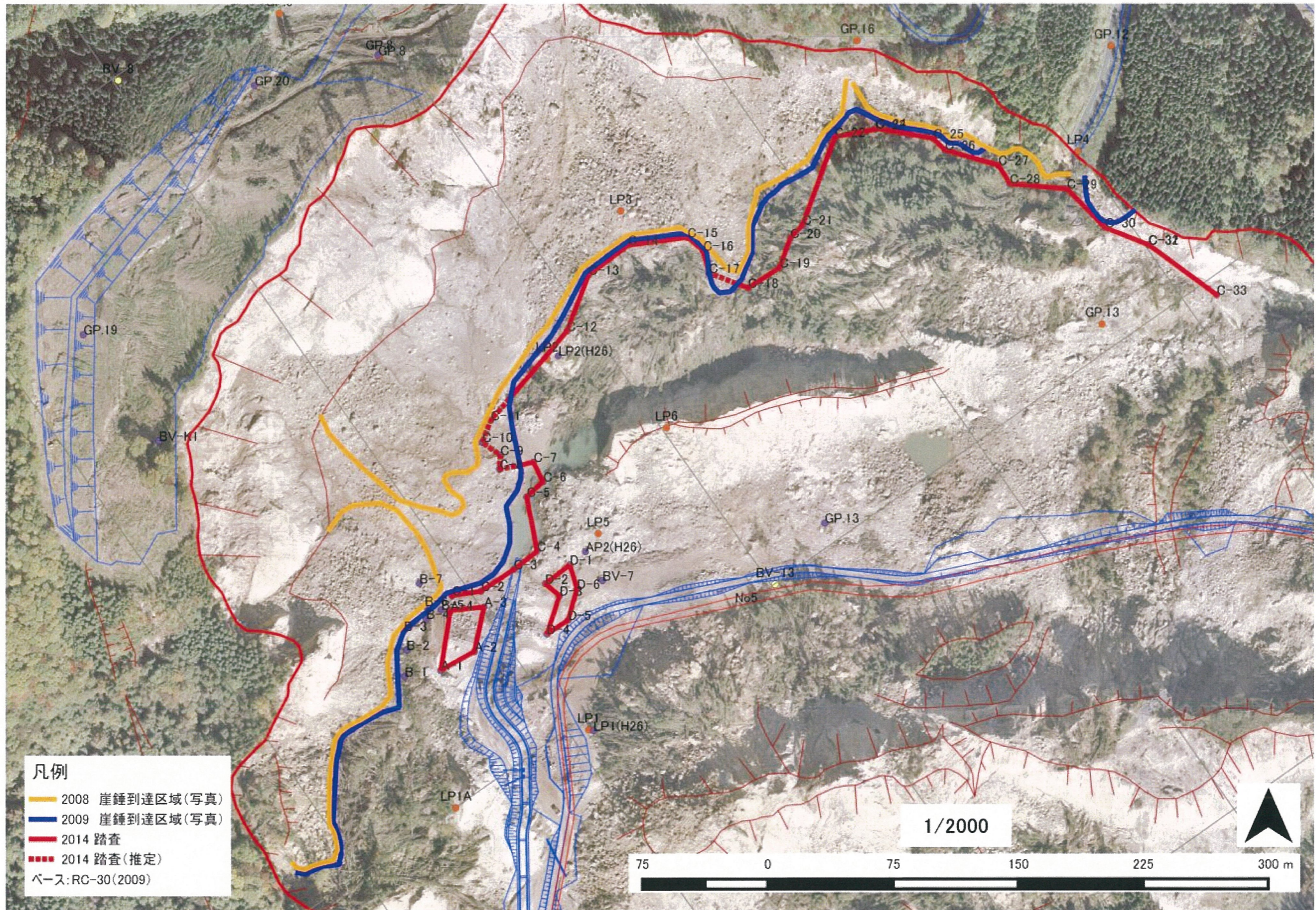
図 2.6.2 RC-30 (2009) / 踏査 (2014) 結果の比較
