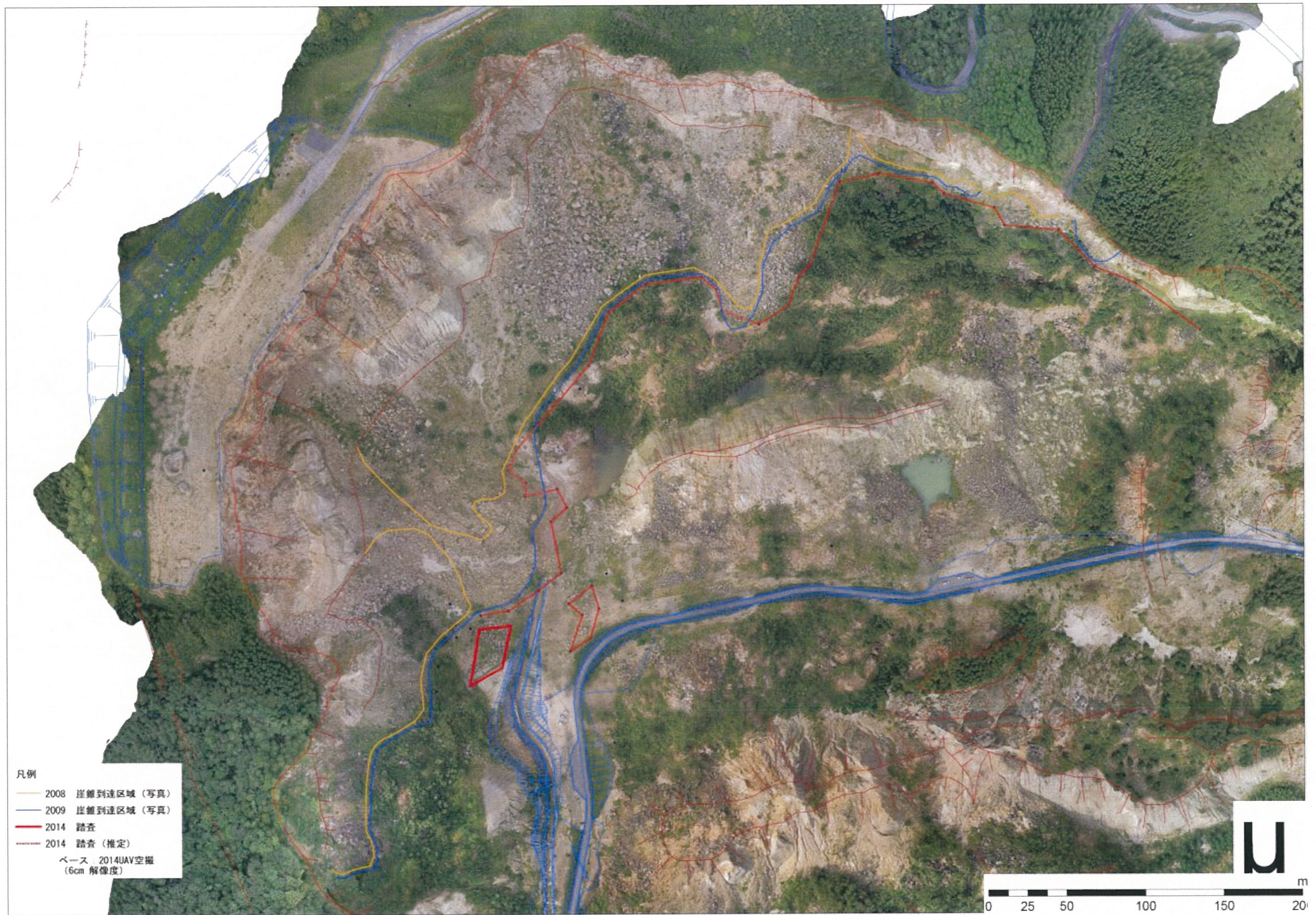
図 2.6.3 UAV / SfM (2014) / 踏査 (2014) 結果の比較
