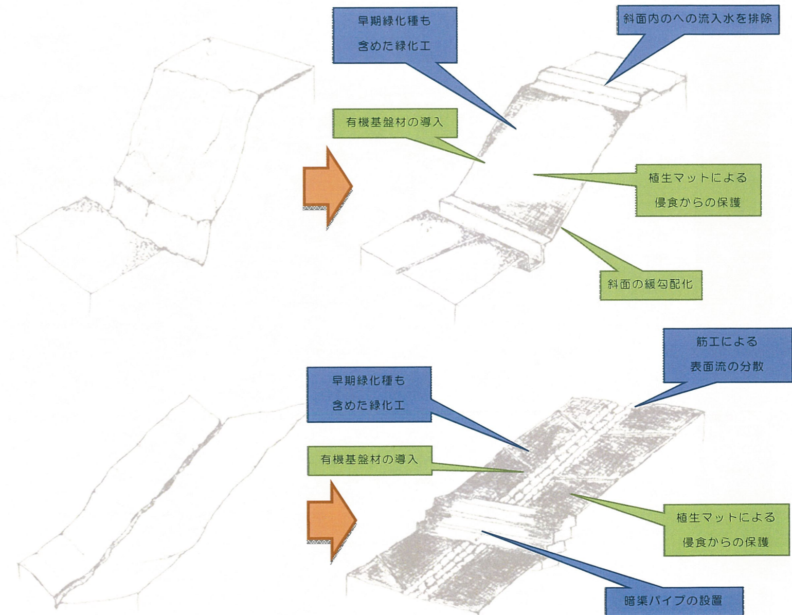
図 2. 5.20 対策（案）概念図
