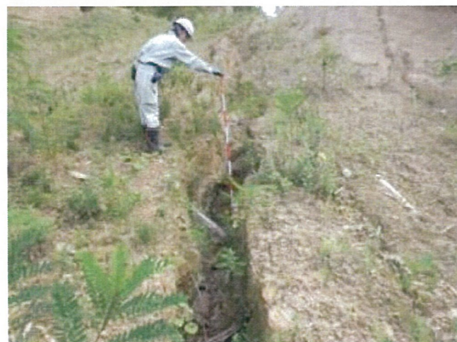
写真 2. 5. 6 集水井下斜面のガリー侵食
