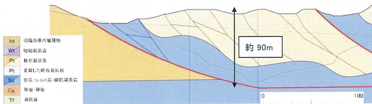
図 2.5.18 荒砥沢地すべり縦断面図
