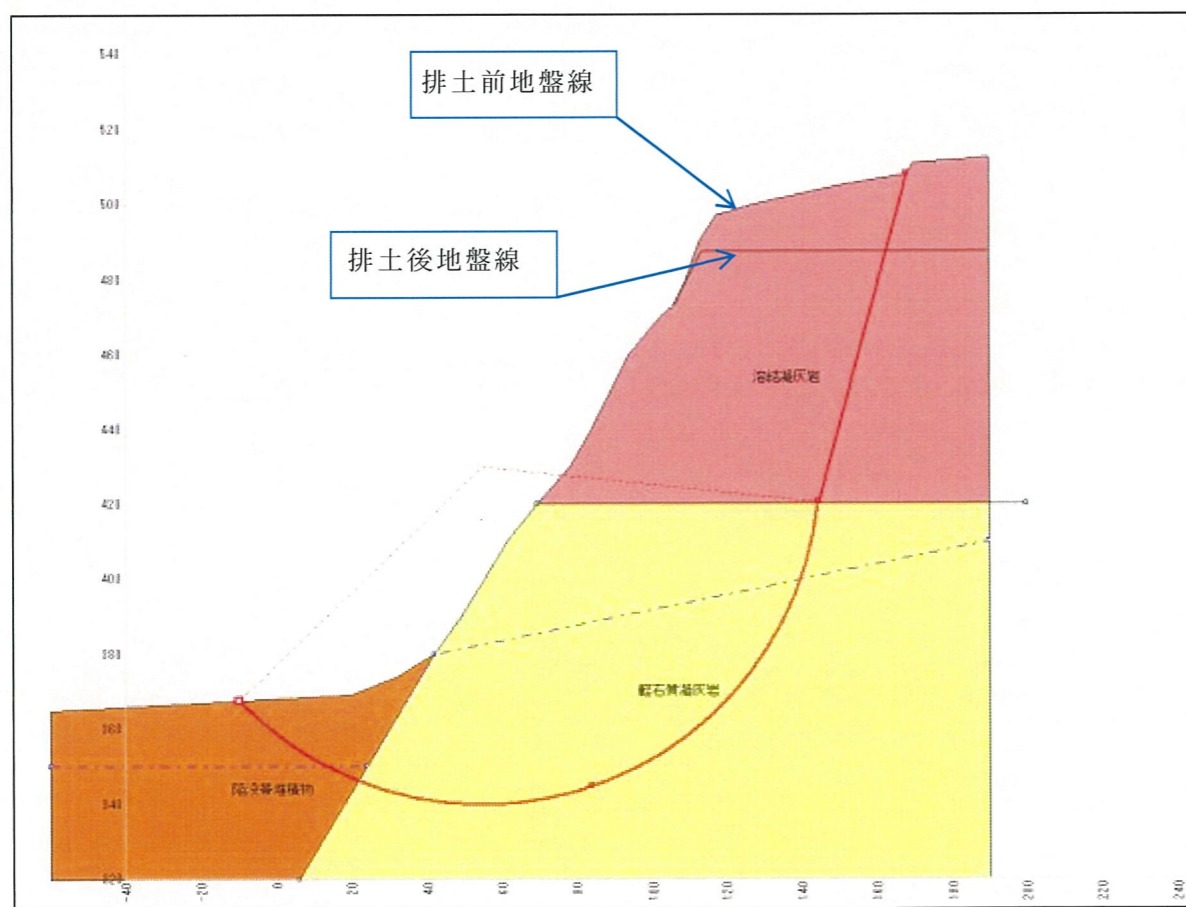
図 2. 4. 28 拡大崩壊断面図 (R 測線)
