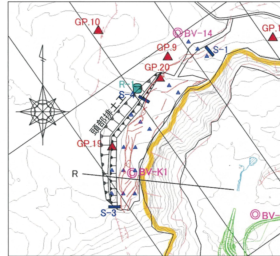
図 2. 4. 25 測線位置図
