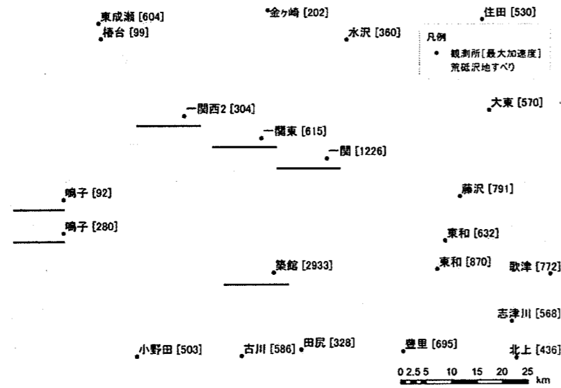
図 2. 4. 31 荒砥沢地すべりと観測所 [最大加速度] の関係 (荒砥沢地すべり周辺拡大図)
