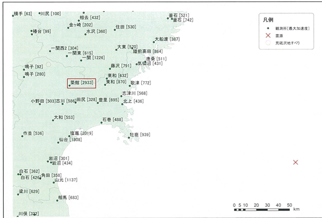
図 2. 4. 23 荒砥沢地すべりと観測所 [最大加速度] の関係
