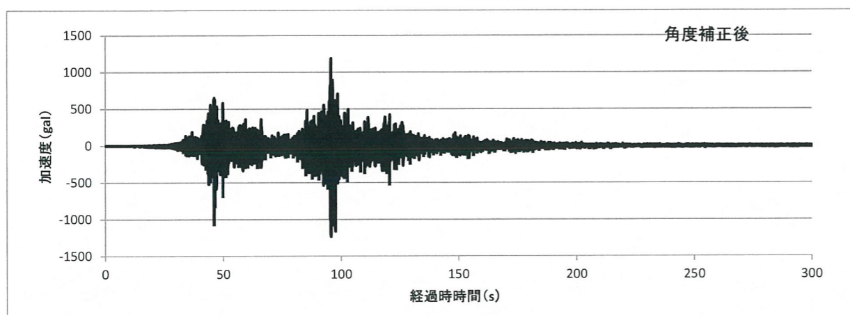
図 2. 4. 27 角度補正後の地震波
