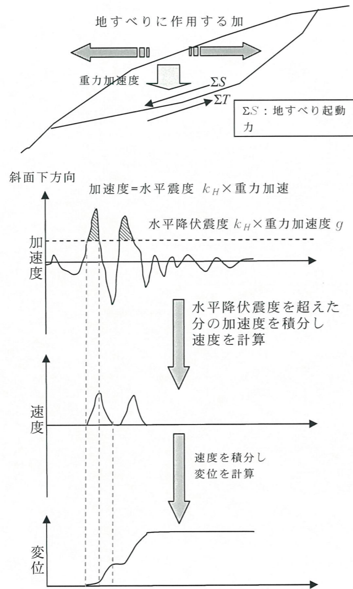
図 2. 4. 29 ニューマーク法の概要
