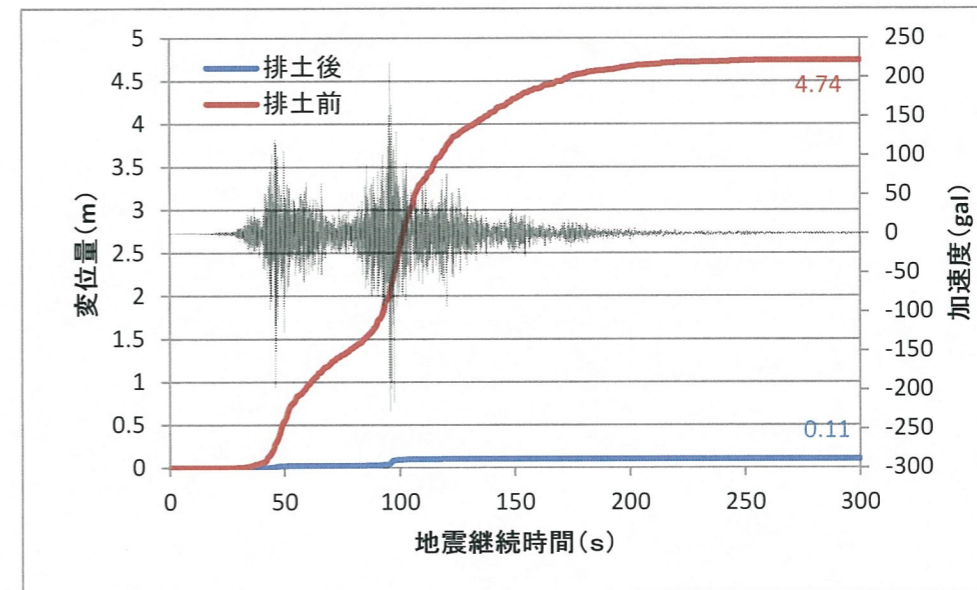
図 2. 4. 30 計算結果 (排土前後の比較)
