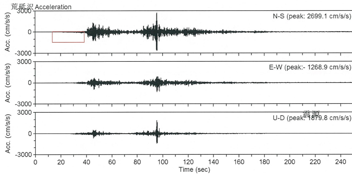
図 2. 4. 24 加速度時刻歴 2011/3/11 14:46 [築館 (MYG004)]
