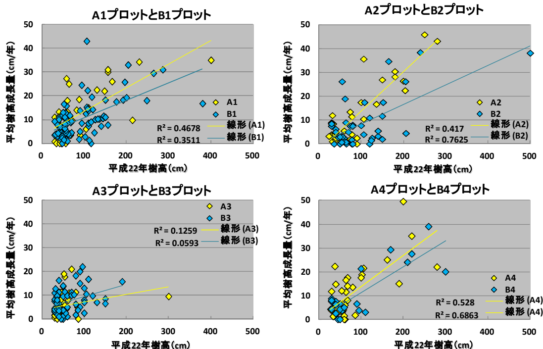
図-4. ヒバ天然稚幼樹の樹高と樹高成長量の関係(4年間)
