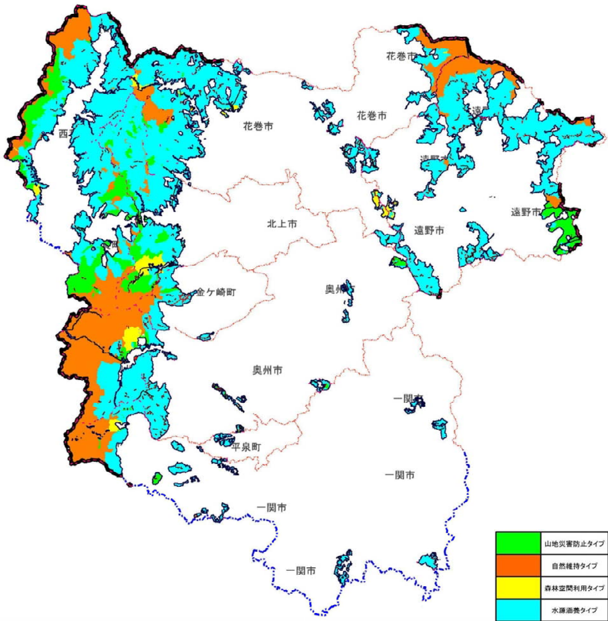
図－2 国有林の機能類型別森林分布図
