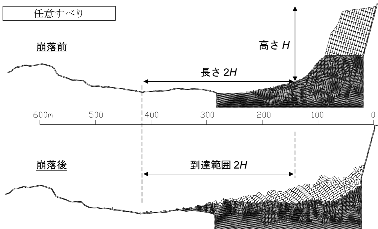
図 3.2.5 計算結果 (任意すべり)
