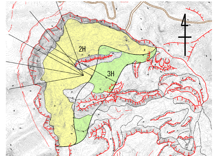
図 3.2.6 到達距離 2H および 3H の範囲
