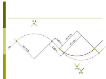
林業専用道の設計
