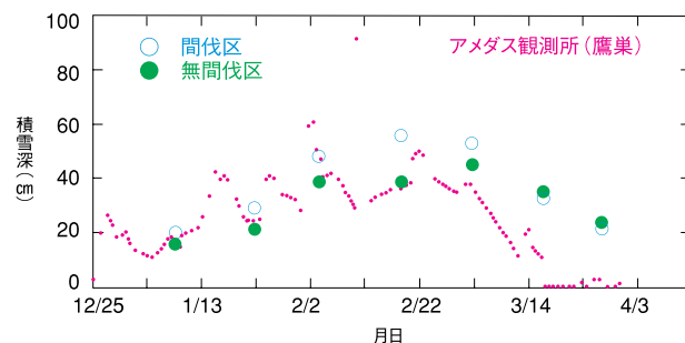
図2 間伐が積雪深に及ぼす影響
