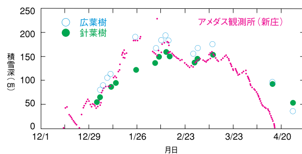
図1 落葉広葉樹林内と常緑針葉樹林内の積雪深の比較
