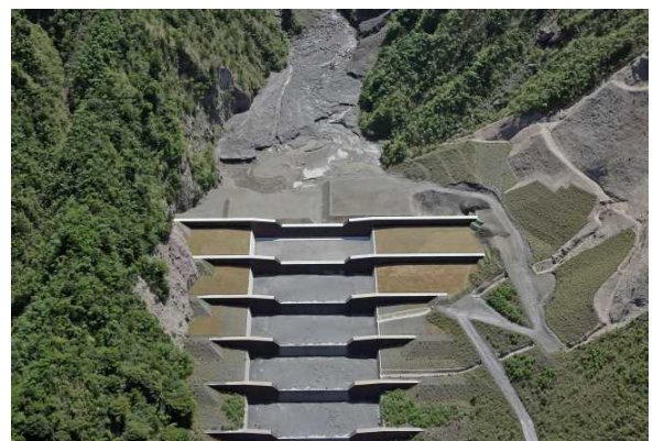
土石流を抑制する溪間工(桜島)
