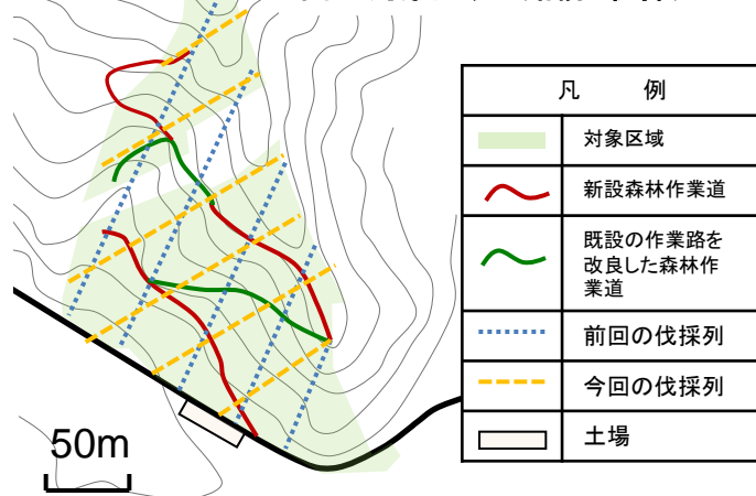
図1:対象区域の路網と伐採列
