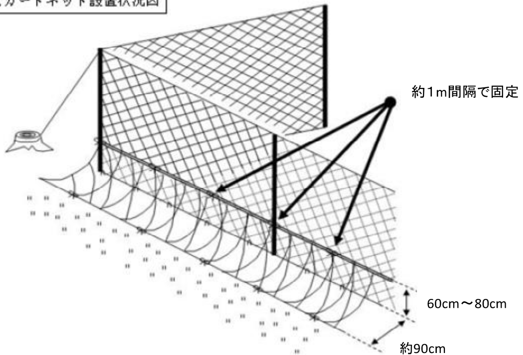
スカートネット設置状況図
