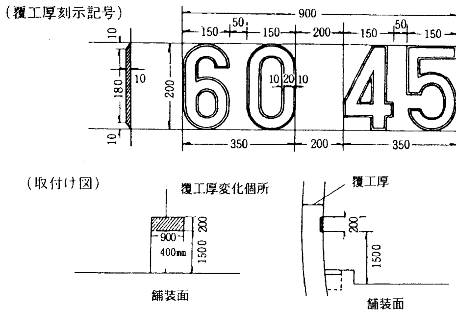
図10-1 覆工厚刻示
