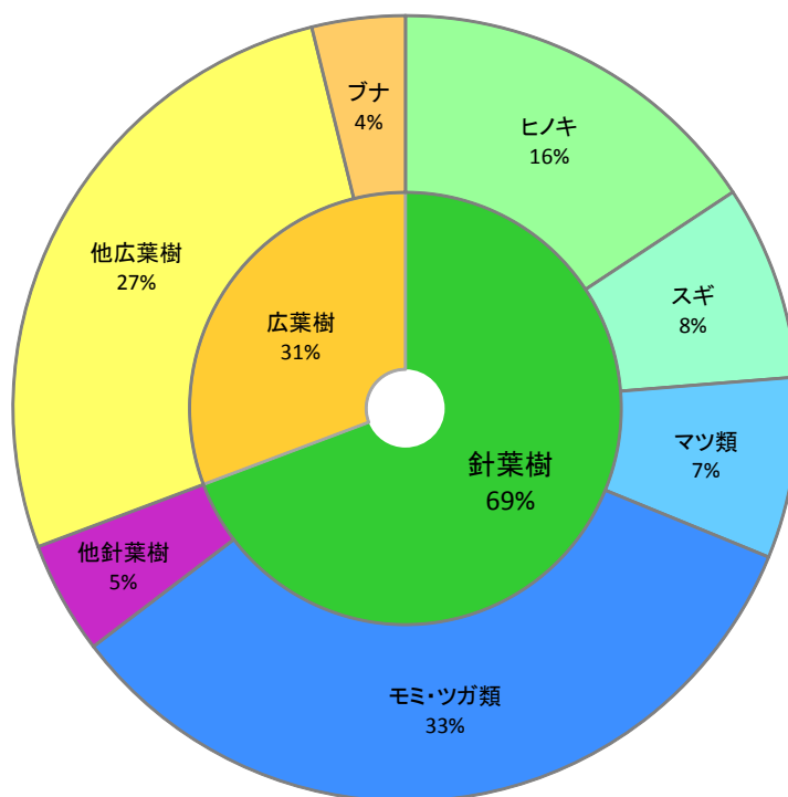
図－2 主な樹種構成（材積比）
