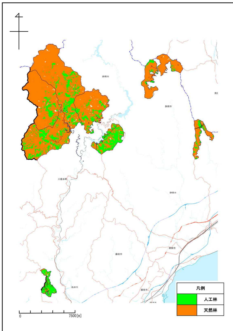
図－１－２ 人工林、天然林の分布状況
