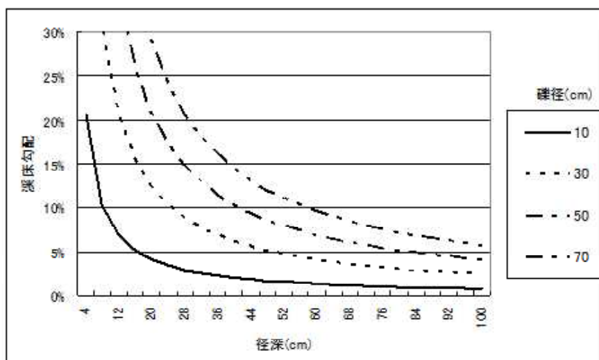
図－５ 石礫の移動する溪床勾配と径深の関係
