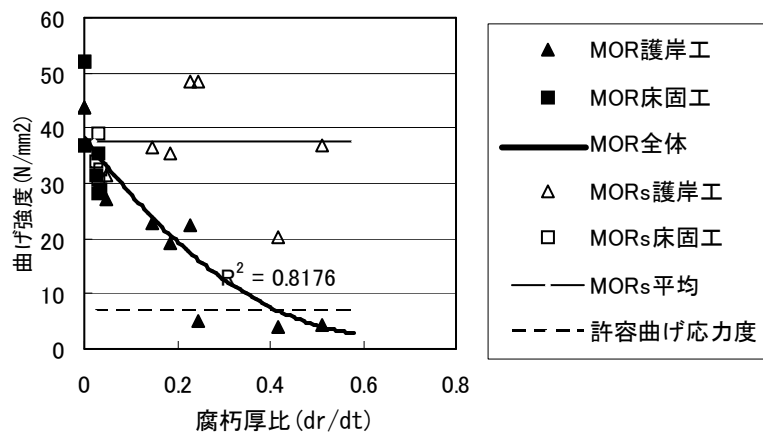
図-3 腐朽厚比( dr/dt )と曲げ強度(MOR, MORs) MORIは全体直径( dt )で計算、MORsは健全部直径( ds )で計算
