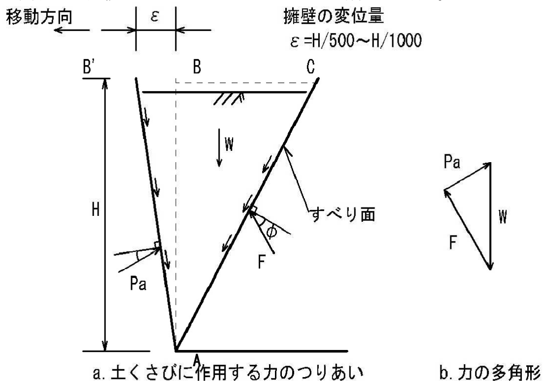
図－１０ クーロンの土くさび
