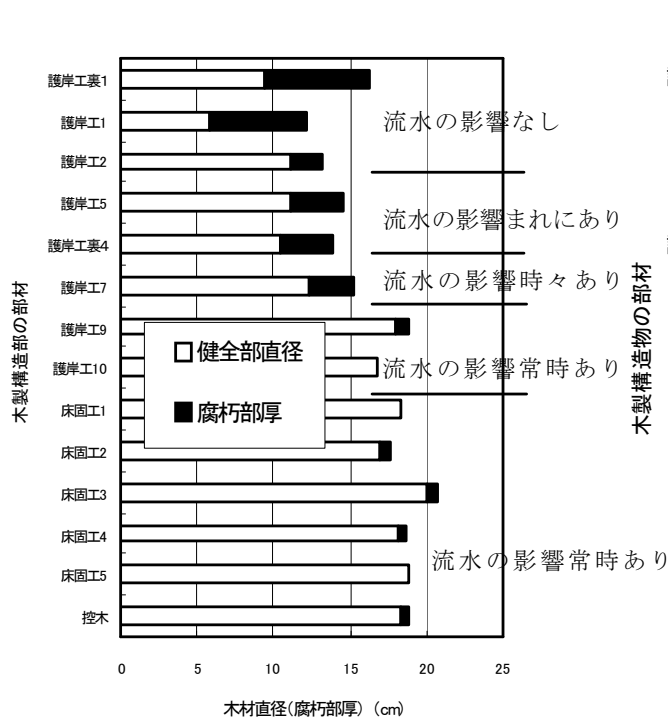
図-1 穿孔抵抗値による健全部直径( d_s )と腐朽厚( d_r )
