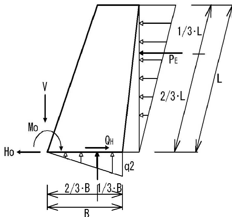
図－９ 地盤反力係数法による簡便法
