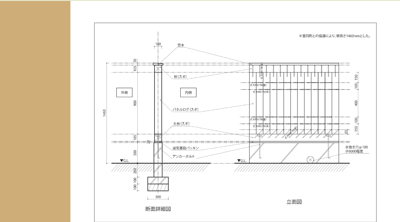
図1 木塀立面図
