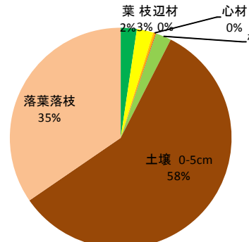
部位別の放射性セシウムの分布割合 (落葉広葉樹二次林)
