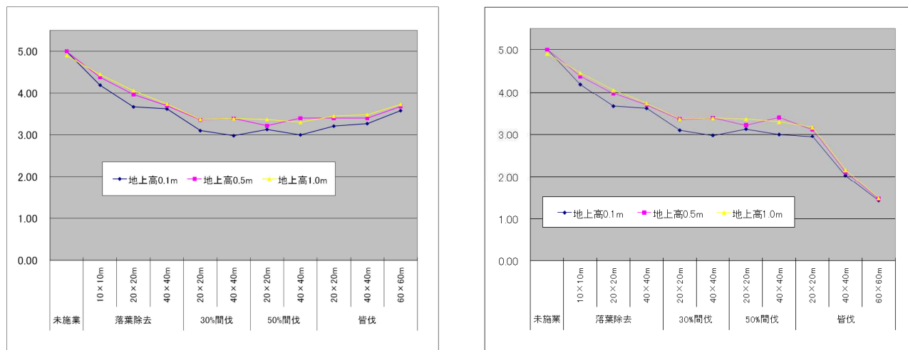
図1 スギ人工林における空間線量率( \mu Sv/h)の変化
