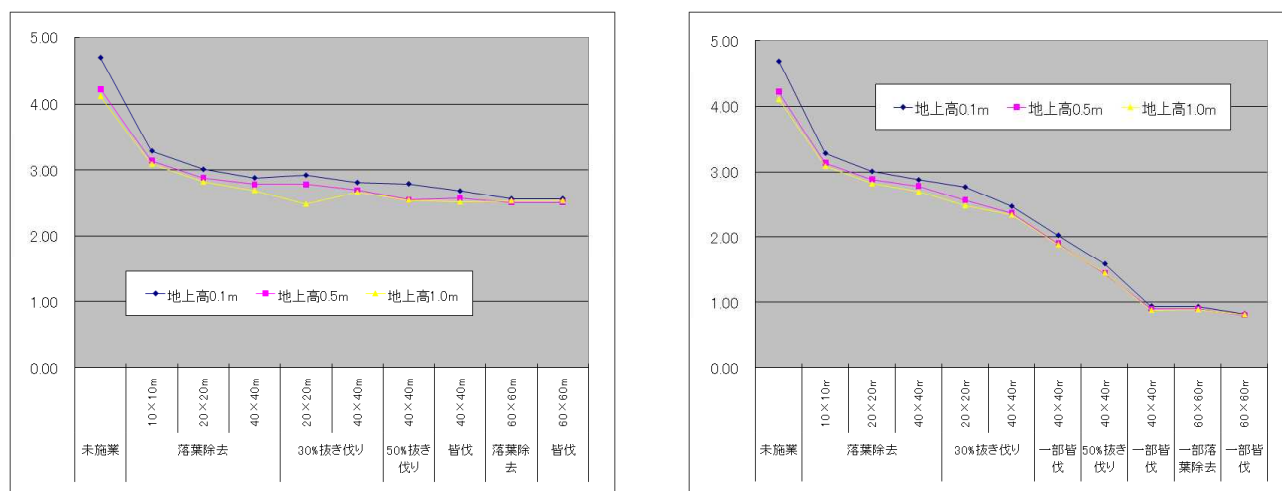
図2 落葉広葉樹林における空間線量率( \mu Sv/h)の変化
