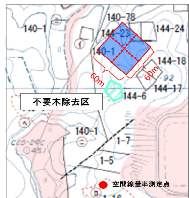
広葉樹二次林
