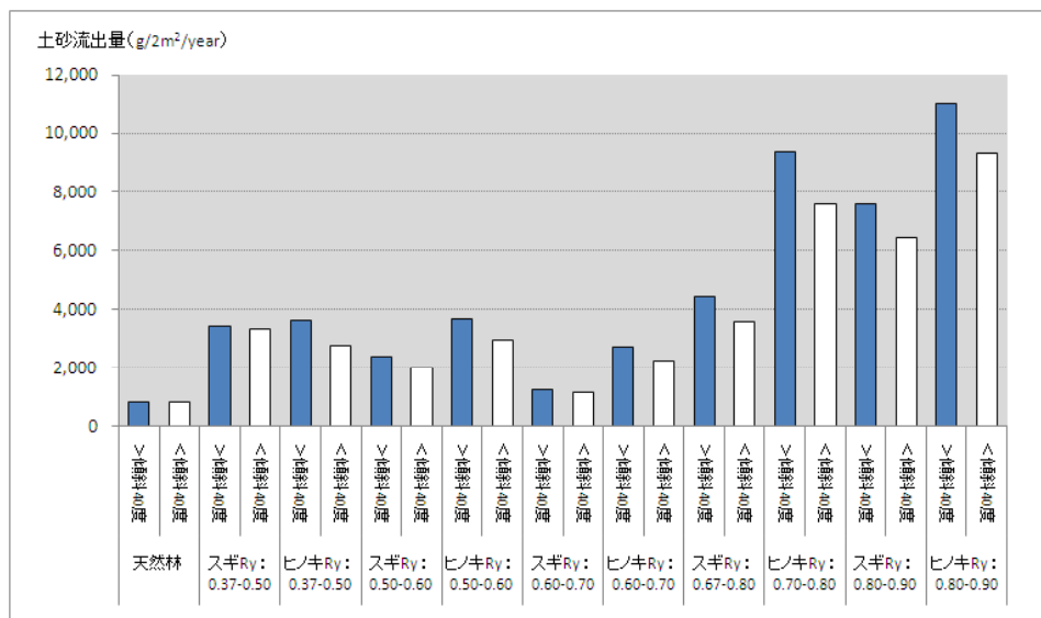
図2 傾斜別・樹種別の収量比数と土砂流出量
