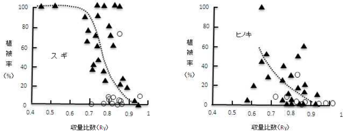
図1 スギ・ヒノキ林内における収量比数と下層植生の植被率
