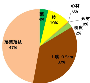
部位別の放射性セシウムの分布割合 (アカマツ・落葉樹混交林)
