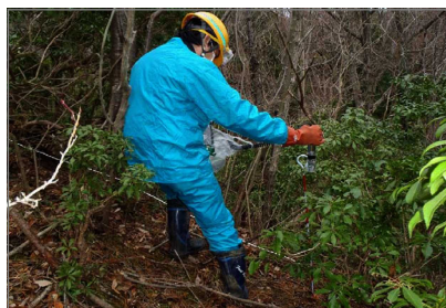
空間線量率の測定 (広葉樹二次林)
