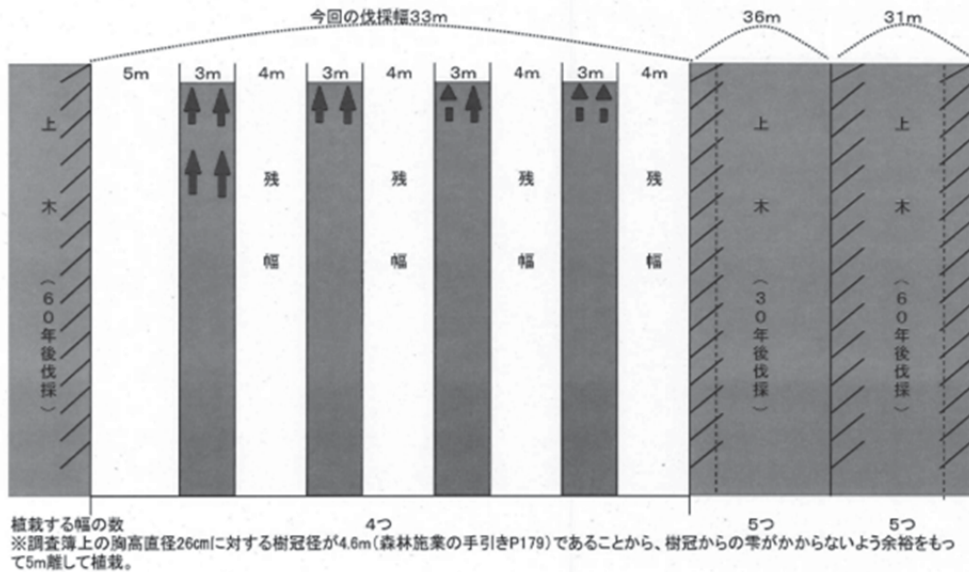
図-3 植栽列模式図
