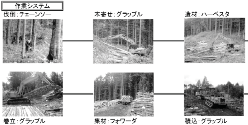
図-2 低コスト高効率作業システム
