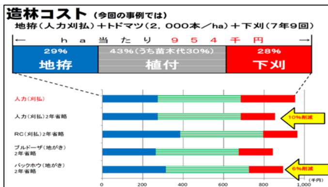
(図4) 下刈省略によるコスト比較
