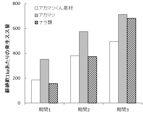
図3 薪絶乾1kgあたりの発生スス量
