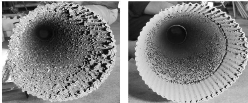
図4. アカマツくん蒸材(左)とナラ類(右)の煙突断面
