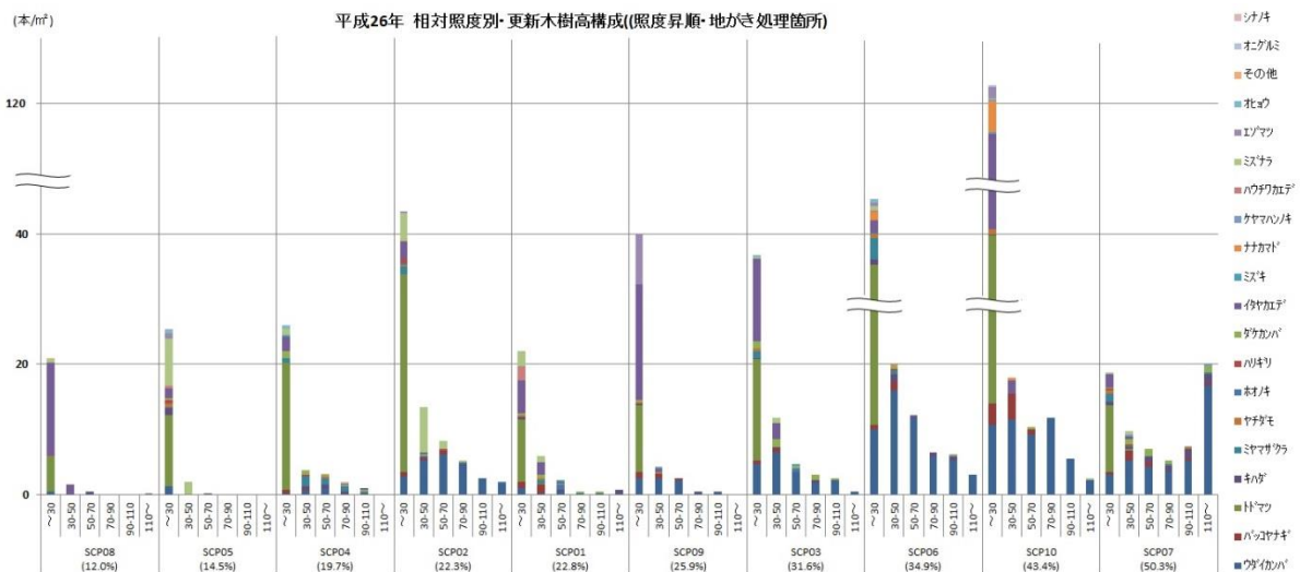
グラフ6 地がき箇所 更新・生存数(光強度/樹高階級順・1 m 2 あたり本数)
