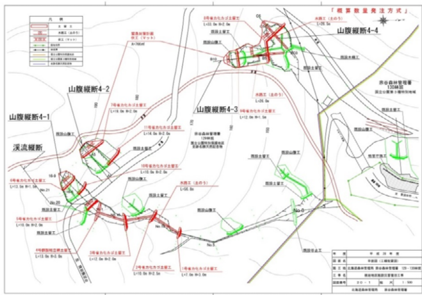
第8・9号土留工
