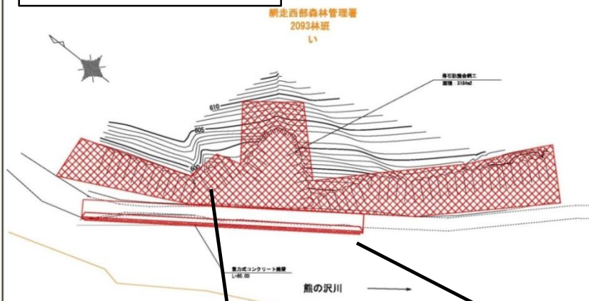
計画(落石防護金網工、擁壁工)
