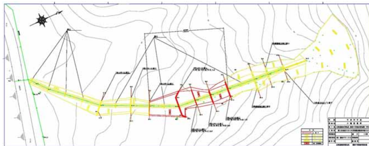
第4号:施工(背面)完了 (H29. 11.30現在)
