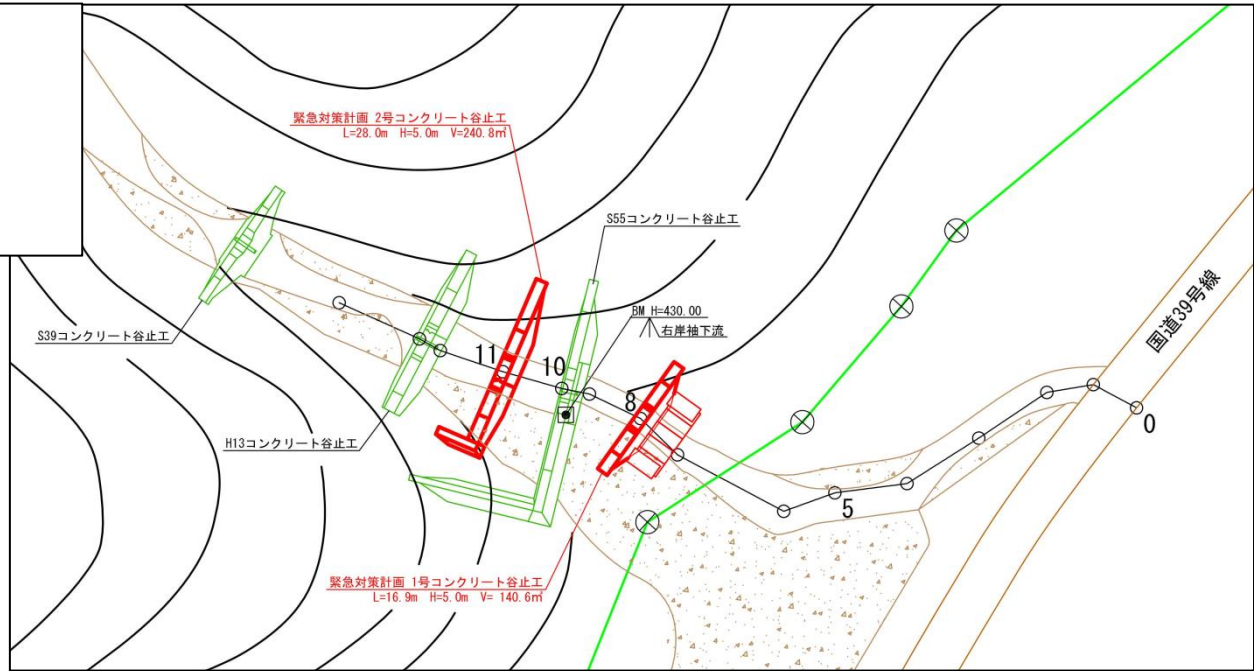
第2号谷止工 (H29.11.21現況)
