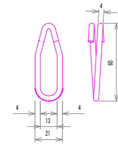
ネット接続金具 S=1:2
