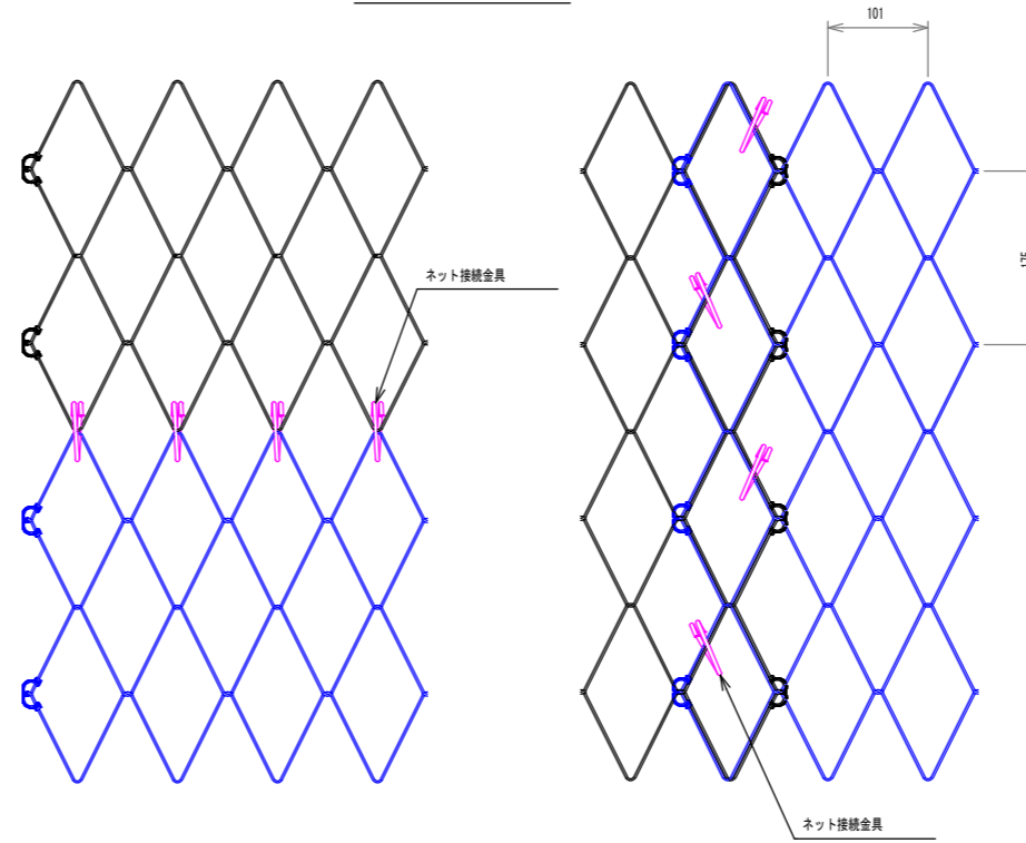
ネット接続例 S=1:6
