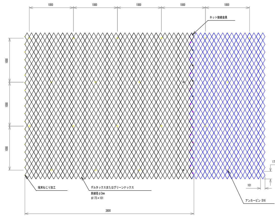
正面図 S=1:30
