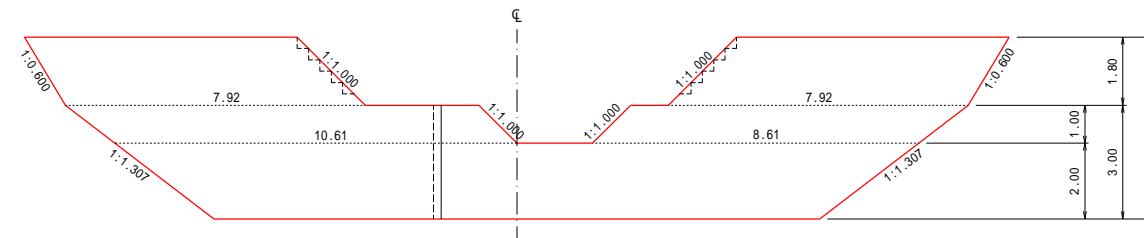
水平打継目(挿筋)計算図 S=1:100
