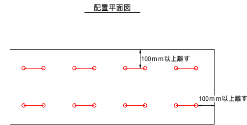
水平打継目標準図 (挿筋)
