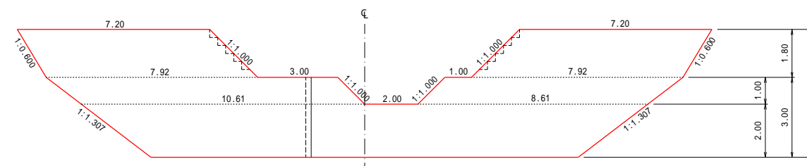
足場工(キヤットワーク)計算図 S=1:100
