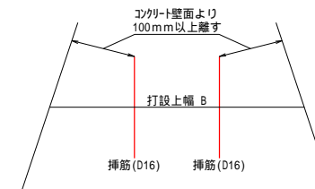
配置側面図
