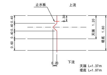
放水路階段詳細図 S=1:50
