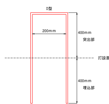
挿筋構造図 D=16mm
