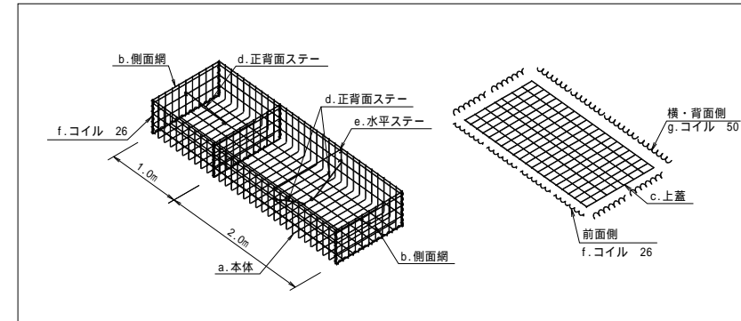
河川用省力化かご工 姿図
