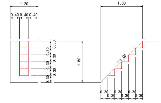
放水路階段詳細図 S=1:50
