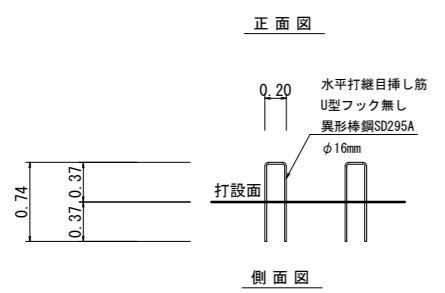
水平打継目挿筋模式図 S=1:50
