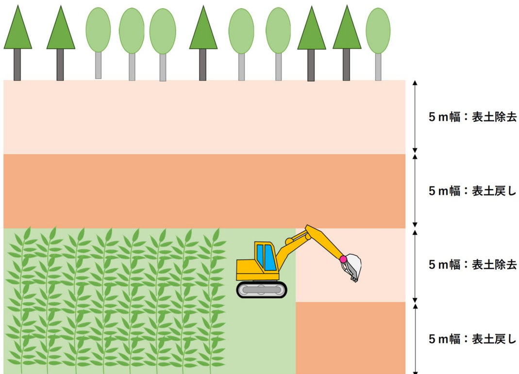
図 表土戻し作業イメージ
