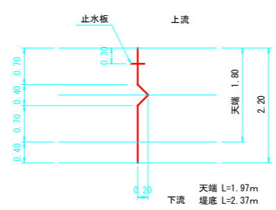
伸縮継目詳細図
