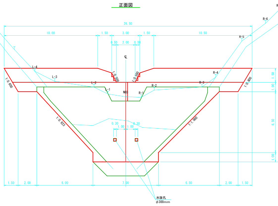
正面図
