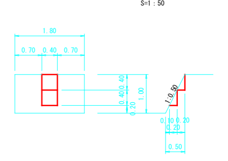
放水路階段詳細図
