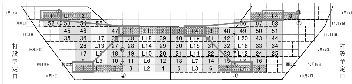
図-3 型枠配置図
