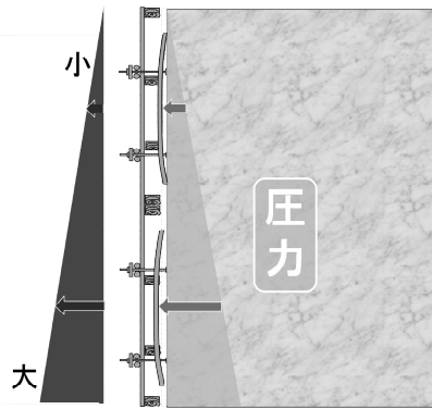
図-15 コンクリート打設よる 型枠合板への圧力
