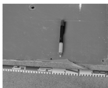
写真-16 塗装面のはがれ
