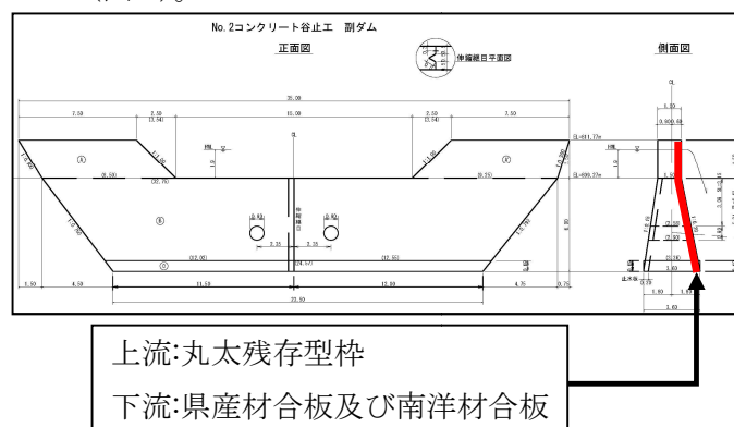
図-2 治山ダム構造図
