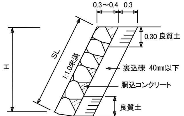
雑石積工(練)
