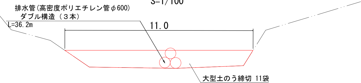
土のう締切計算図 S=1/100
