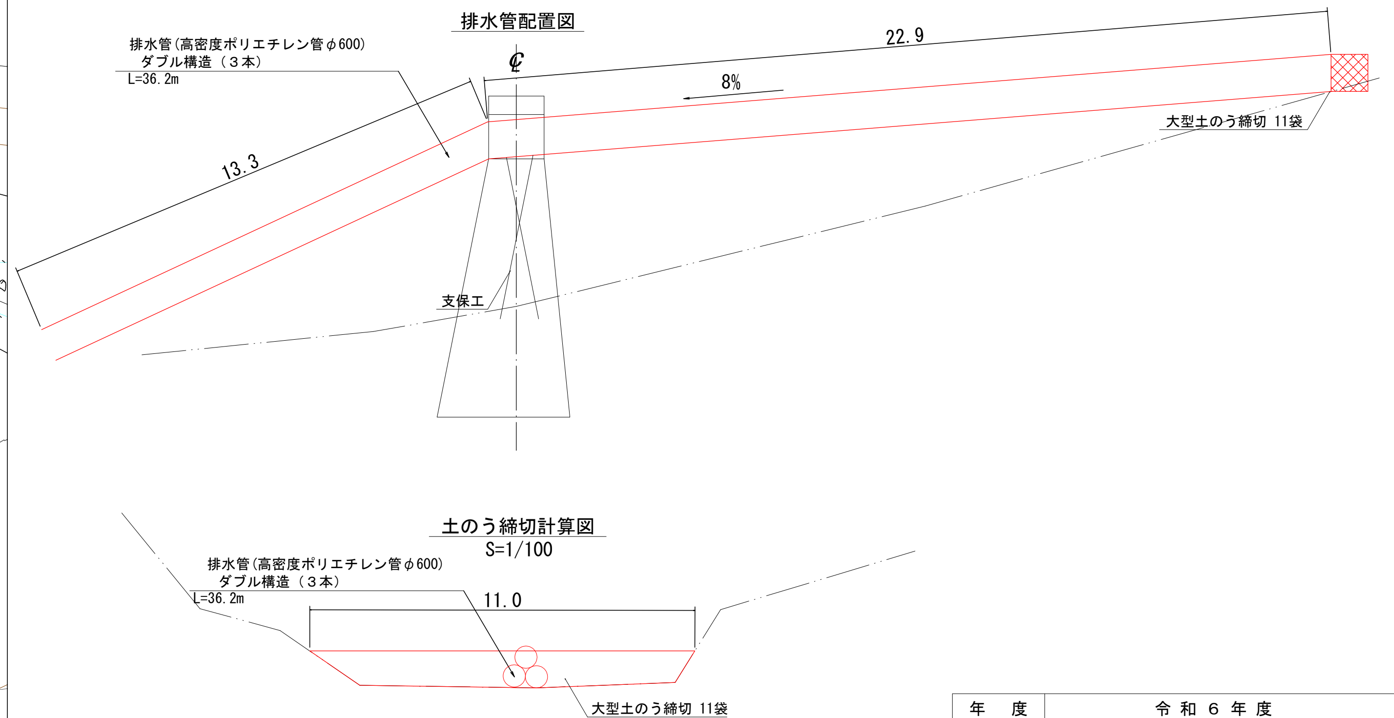
仮締切・廻排水計画図 S=1/100
